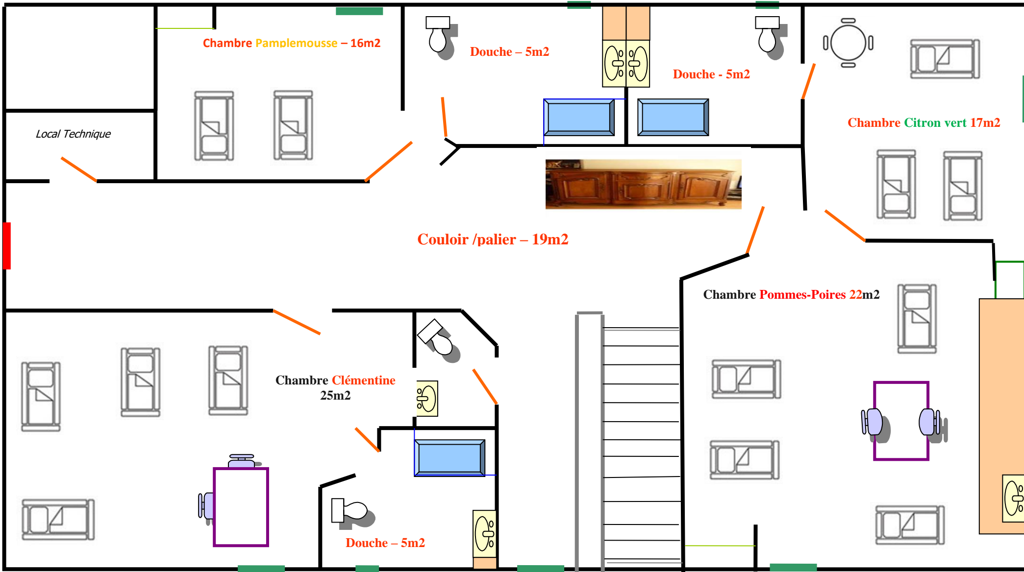
Plan du 1 er étage du Gîte " Clémentine "
